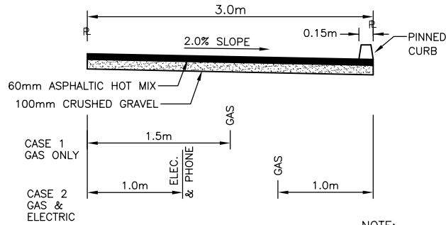
"WALKWAY" N.T.S.
